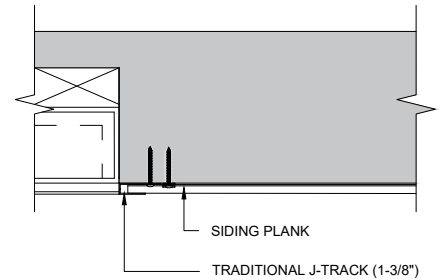
4 JAMB DETAIL SCALE: 1:10
