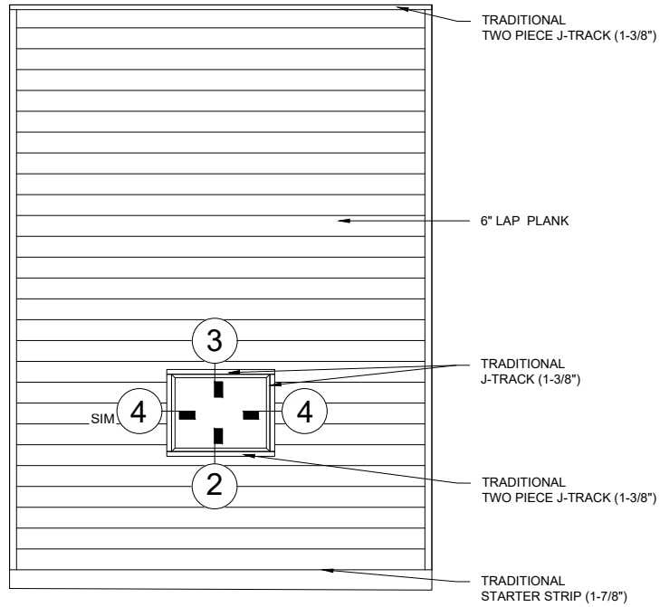
1 WALL ELEVATION SCALE: 1:50
