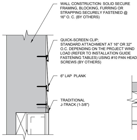
3 HEAD DETAIL SCALE: 1:10
