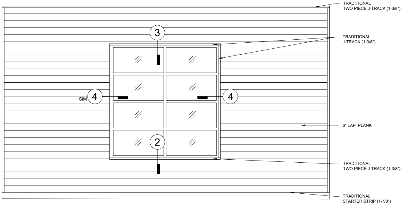
1 WALL ELEVATION SCALE: 1:50
