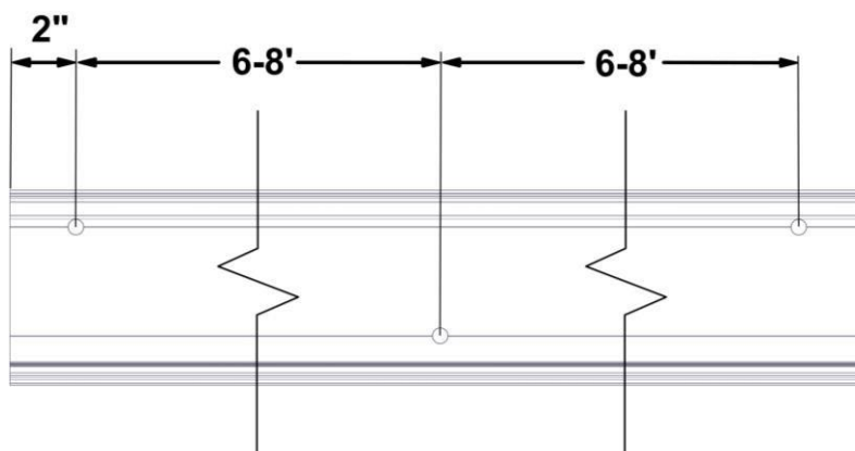
Orientation des tasseaux
