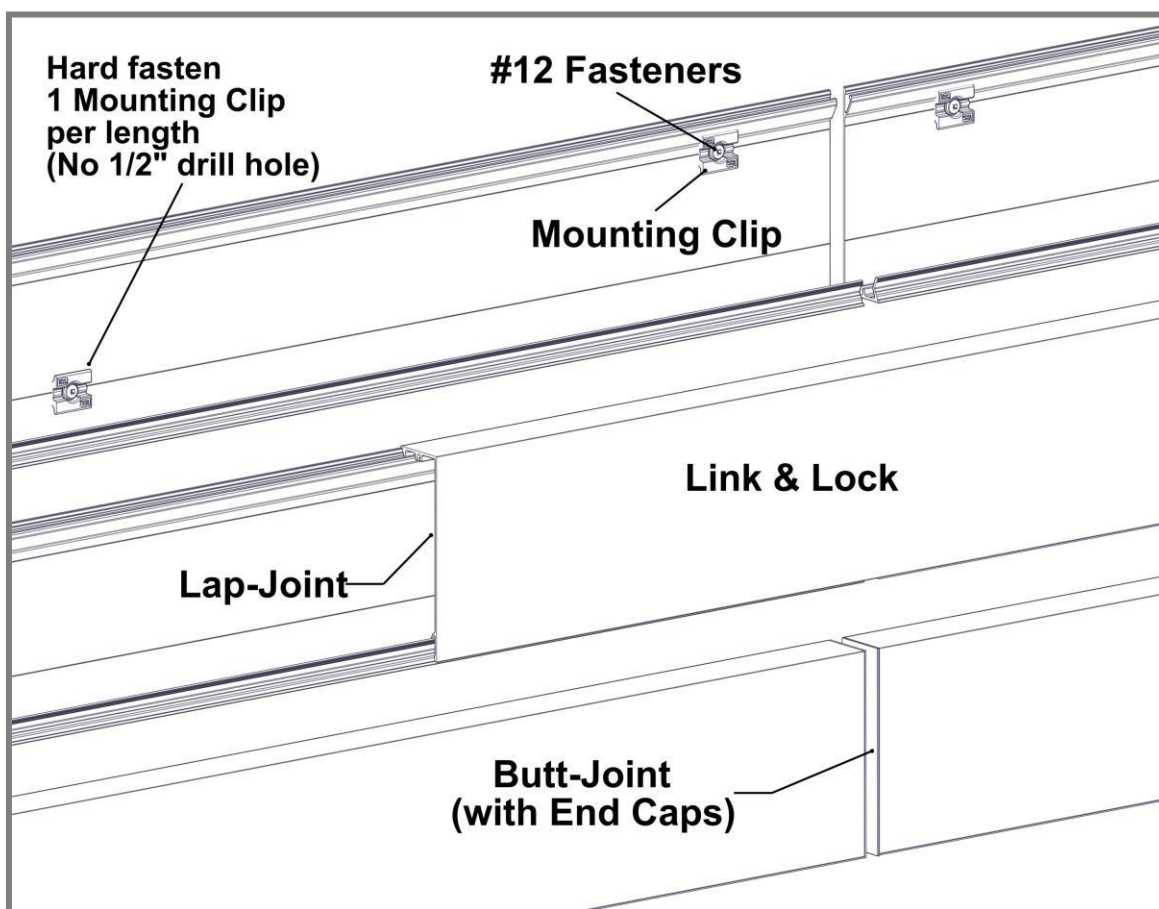
Détail A
